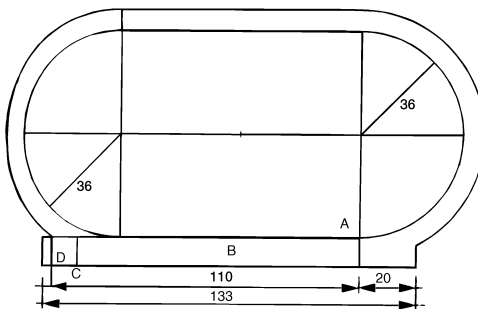
Atletická běžecká dráha: délka 400 m, 6 drah v okruhu, 8 drah v rovině; A start a cíl na 400 a 800 m, B cílová rovinka, C start na 100 m, D start na 110 m překážek
