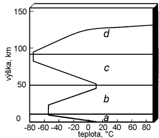
Průběh teploty v atmosféře Země: a troposféra, b stratosféra, c mezosféra, d termosféra, o ozonoféra, i ionosféra
