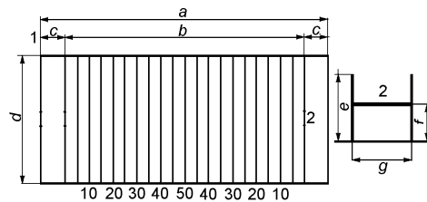
Hřiště na americký fotbal: 1 hřiště, 2 branka; a 120 yardů, b 100 yardů, c 10 yardů, d 53,5 yardů, e 6,1 m, f 3,5 m, g 5,5 m
