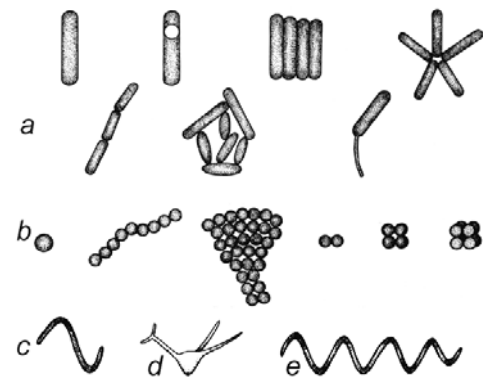
Základní tvary bakterií: a tyčinky, b koky, c spirily, d tvar prostěkatý, e spirochety
